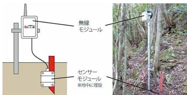
地表傾斜計(感太郎) (中央開発㈱ホームページより転用)
