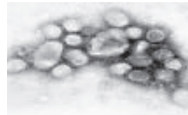
新型インフルエンザ ウイルス H1N1
